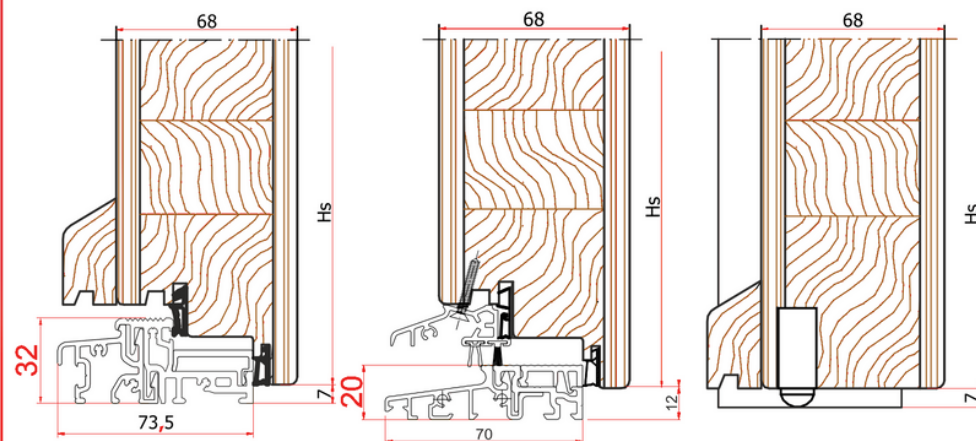
SOGLIA IN ALLUMINIO GUTMANN 74/32 TI
