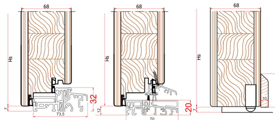
SOGLIA IN ALLUMINIO GUTMANN 74/32 TI
