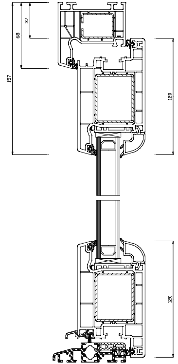
Schnitt S1(5:1)
