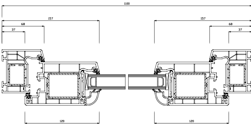
Schnitt S2(5:1)
